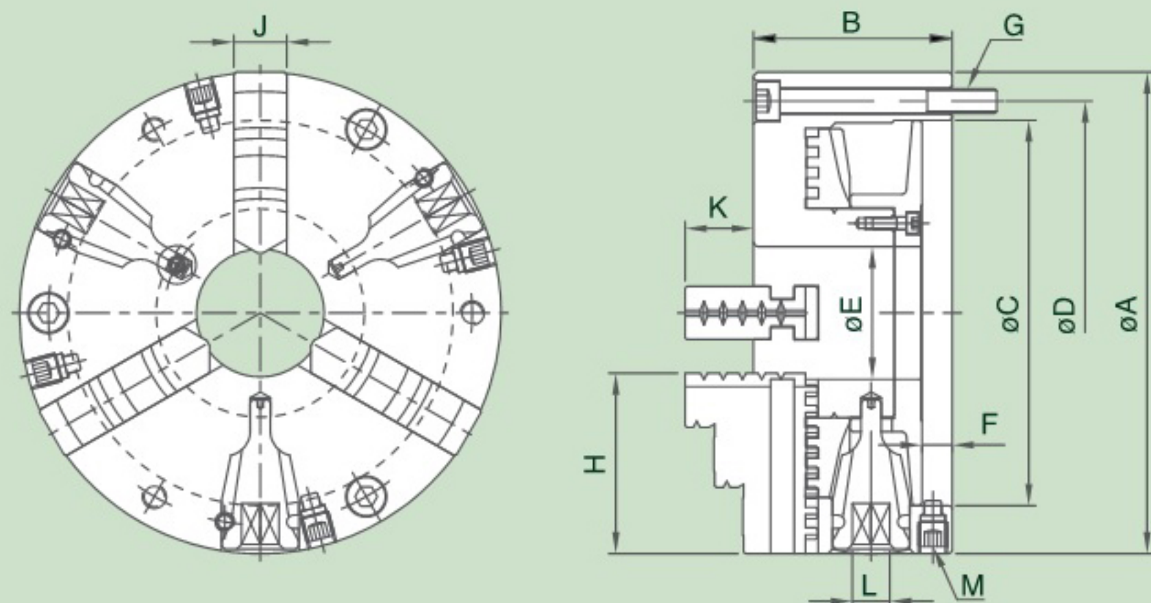
尺寸圖 » Dimensions
